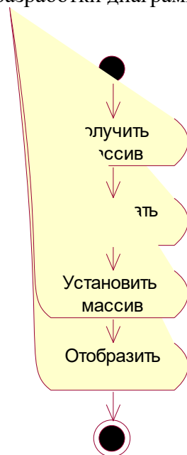
Рис. 39. Диаграмма активности
